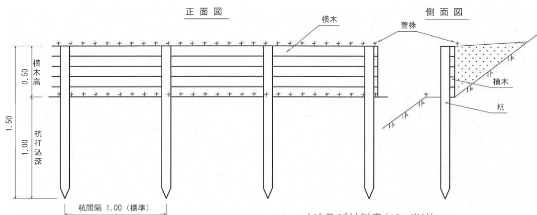
寸法及び材料表(10m当り)
