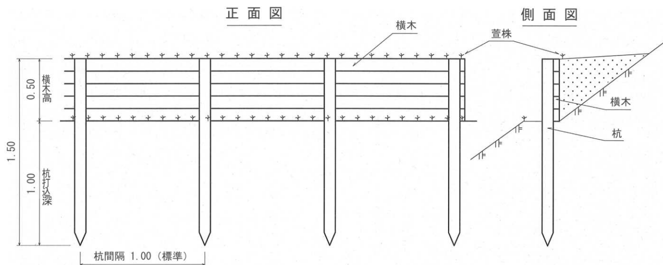
寸法及び材料表(10m当り)
