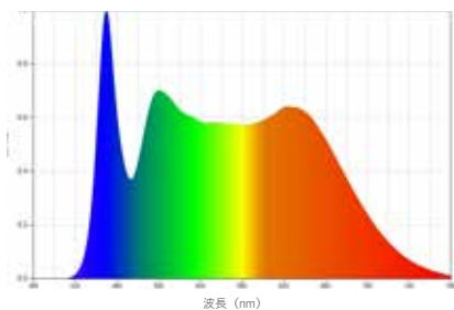
使用 LED の分光スペクトル
